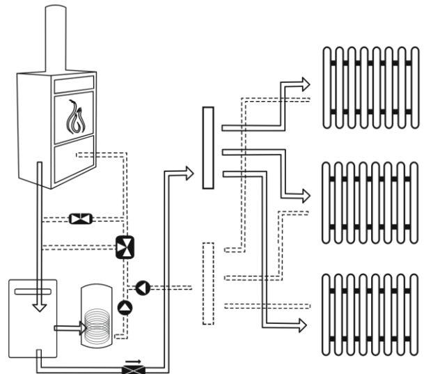
Chaudière à gaz/mazout avec ECS
