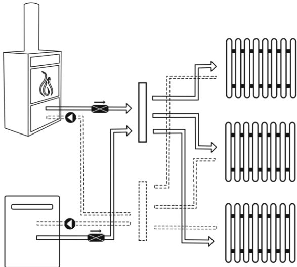
Chaudière à gaz/mazout sans ECS
